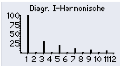
Abbildung 75 Diagramm I-Harmonische, 100%
