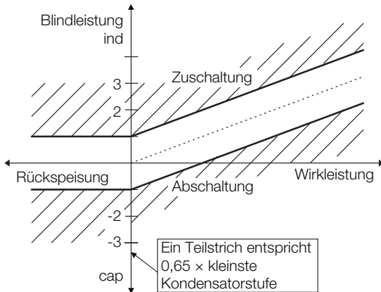
Abbildung 46 Regelverhalten bei \cos \varphi_{\text{soll}} = 0,92 ind; Begrenzung = 0; Parallelverschiebung = 0
