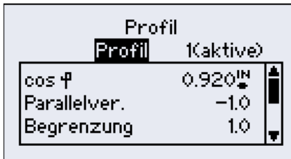
Abbildung 43 Reglerprofil Parameter (Profil ändern) Abbildung 44 Reglerprofil parametrieren
