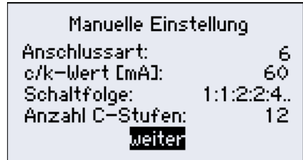
Abbildung 22 Erkennung: Manuell Untermenü
