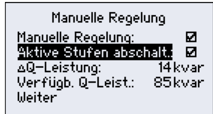
Abbildung 35 Manuelle Regelung Stufenabschaltung
